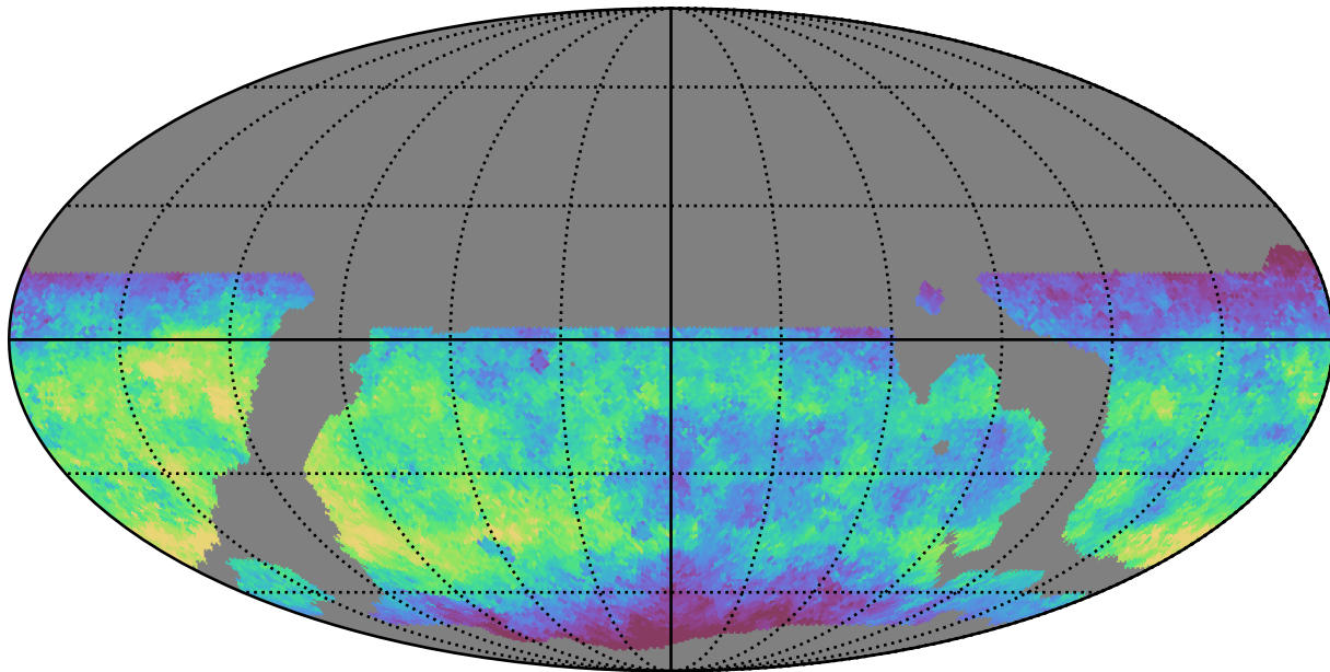
weather_cloudso18v3.4_10yrs WFD g band: Median saturation_mag
