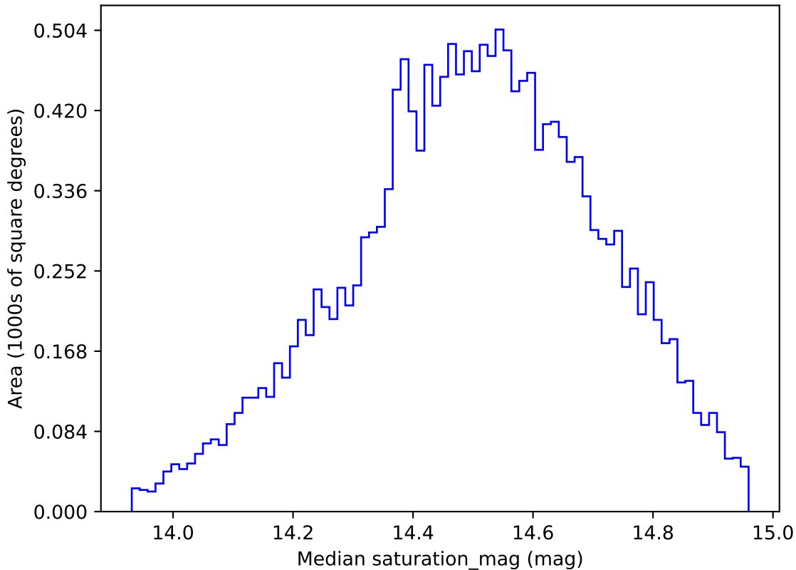
weather_cloudso18v3.4_10yrs WFD g band: Median saturation_mag
