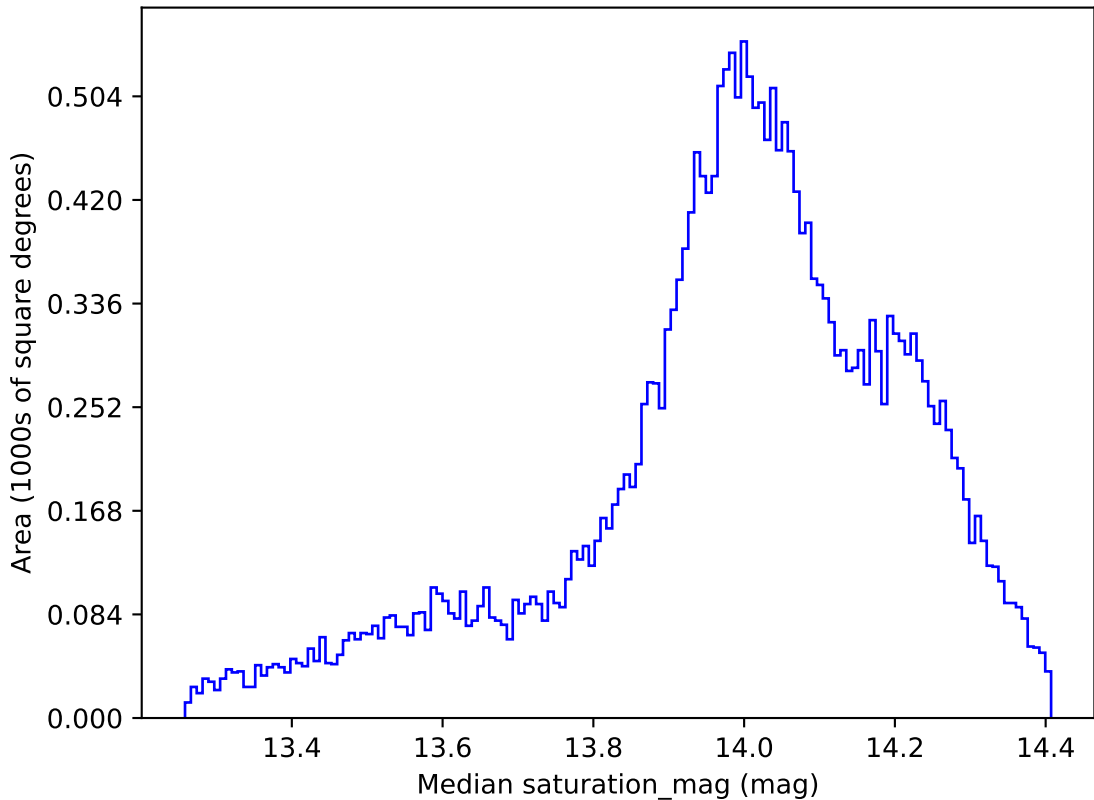
weather_cloudso18v3.4_10yrs All sky z band: Median saturation_mag
