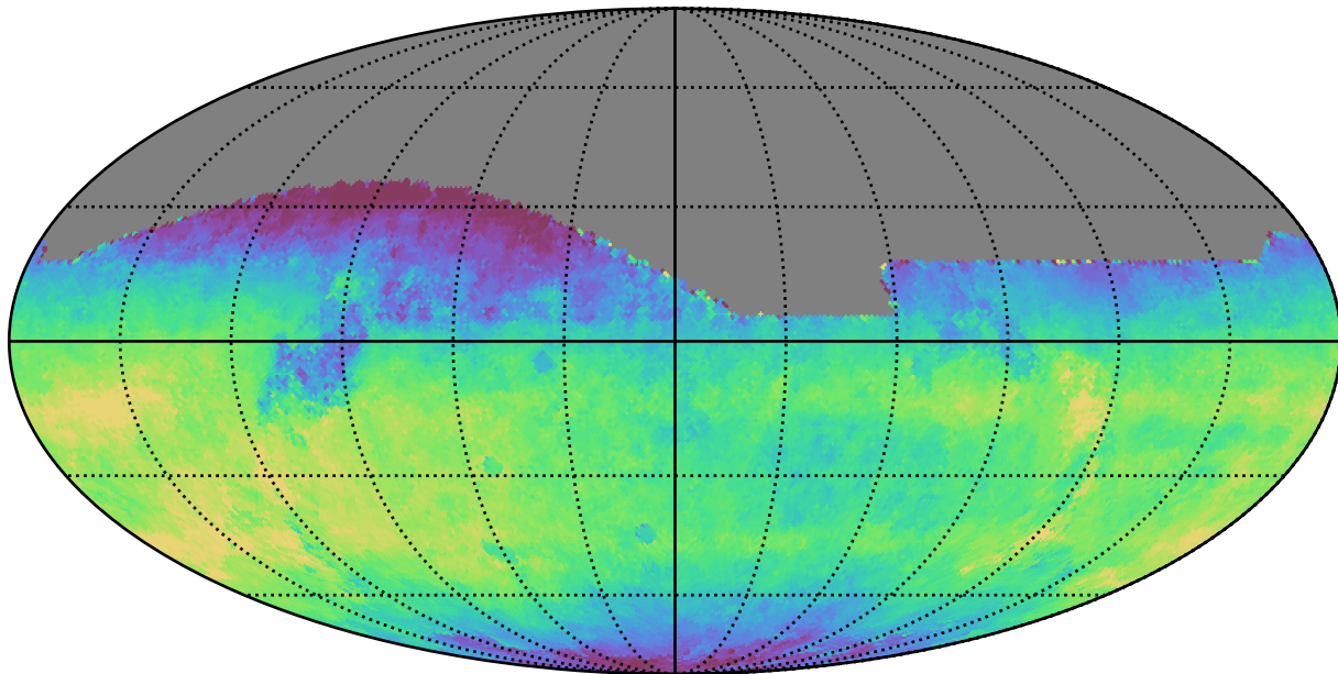
weather_cloudso18v3.4_10yrs All sky r band: Median saturation_mag
