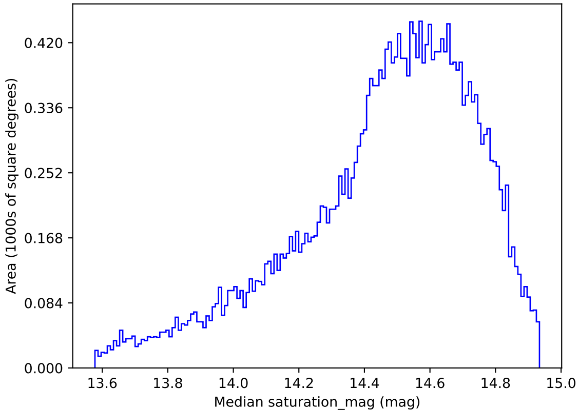
weather_cloudso18v3.4_10yrs All sky r band: Median saturation_mag
