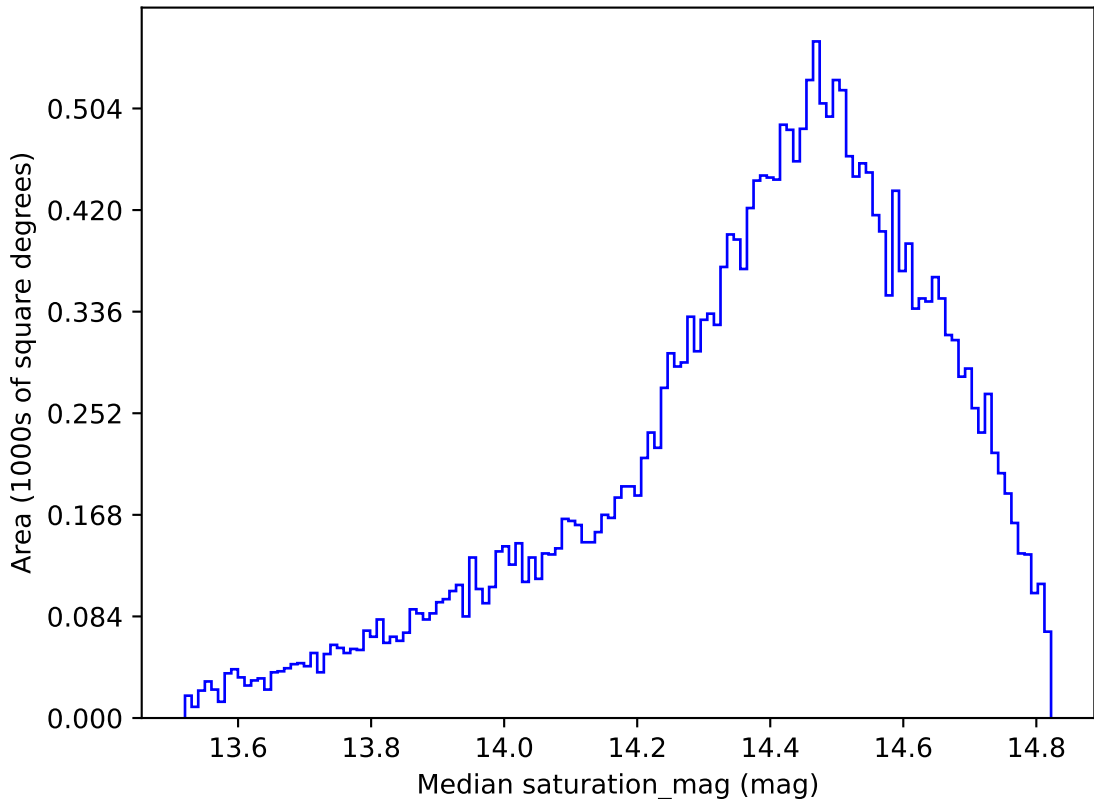
weather_cloudso18v3.4_10yrs All sky i band: Median saturation_mag
