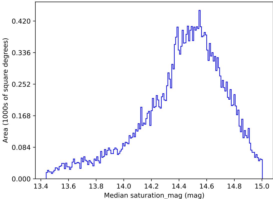
weather_cloudso18v3.4_10yrs All sky g band: Median saturation_mag
