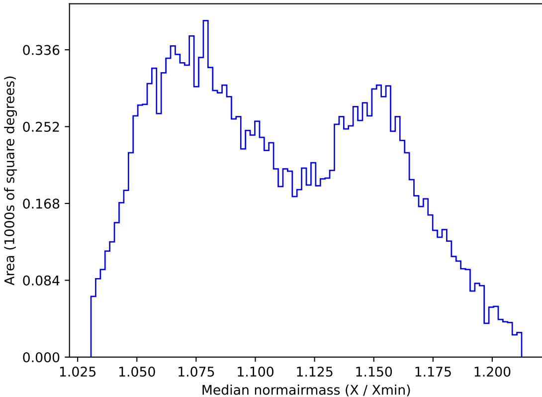
weather_cloudso18v3.4_10yrs WFD y band: Median normairmass
