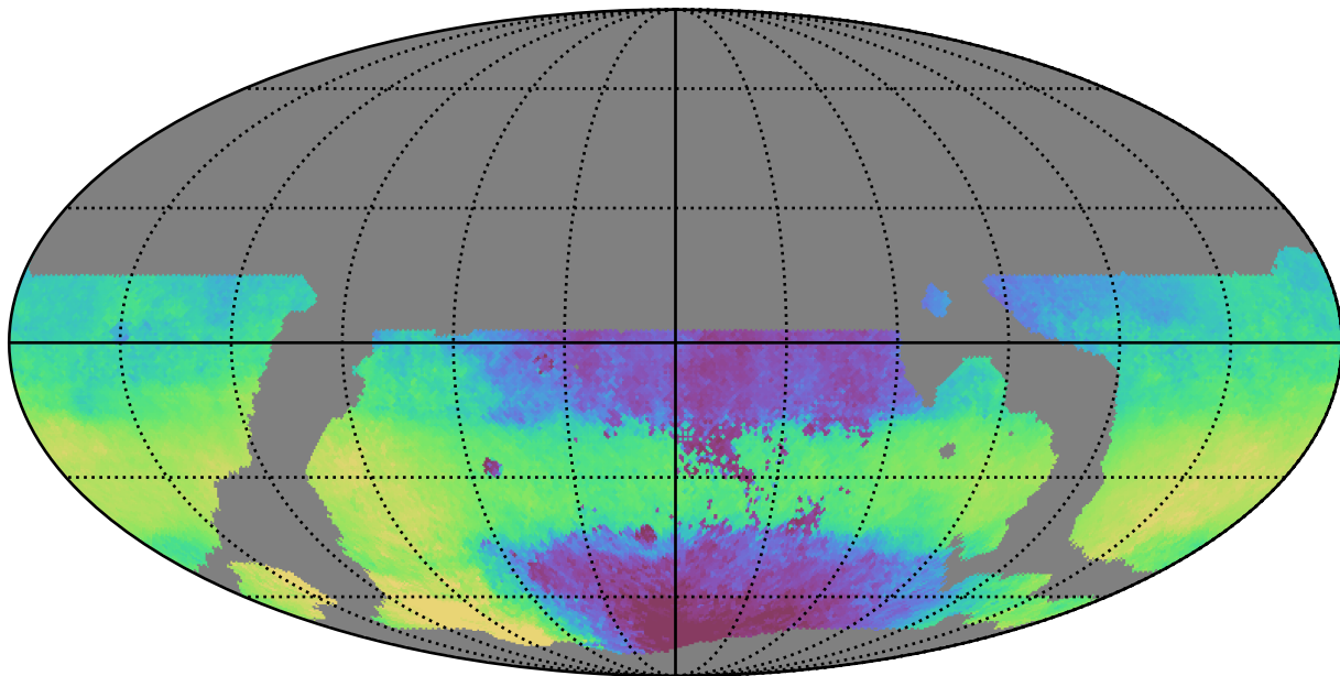
weather_cloudso18v3.4_10yrs WFD y band: Median HA
