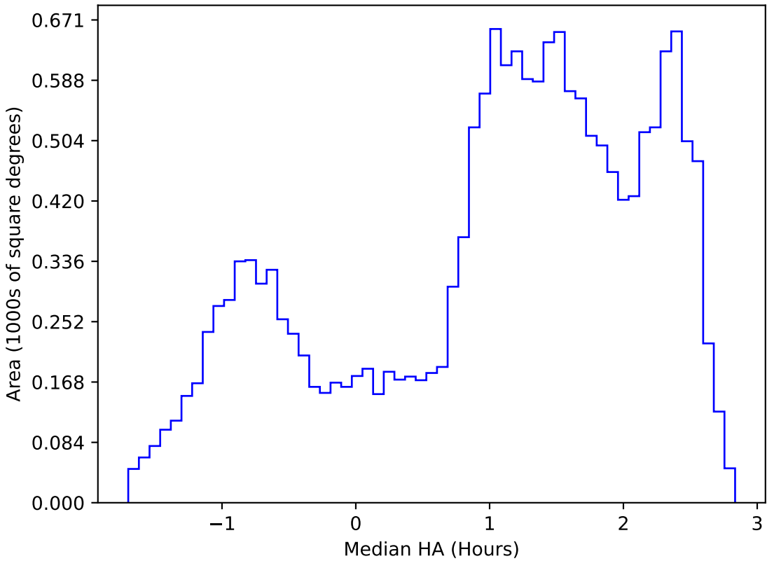
weather_cloudso18v3.4_10yrs WFD y band: Median HA
