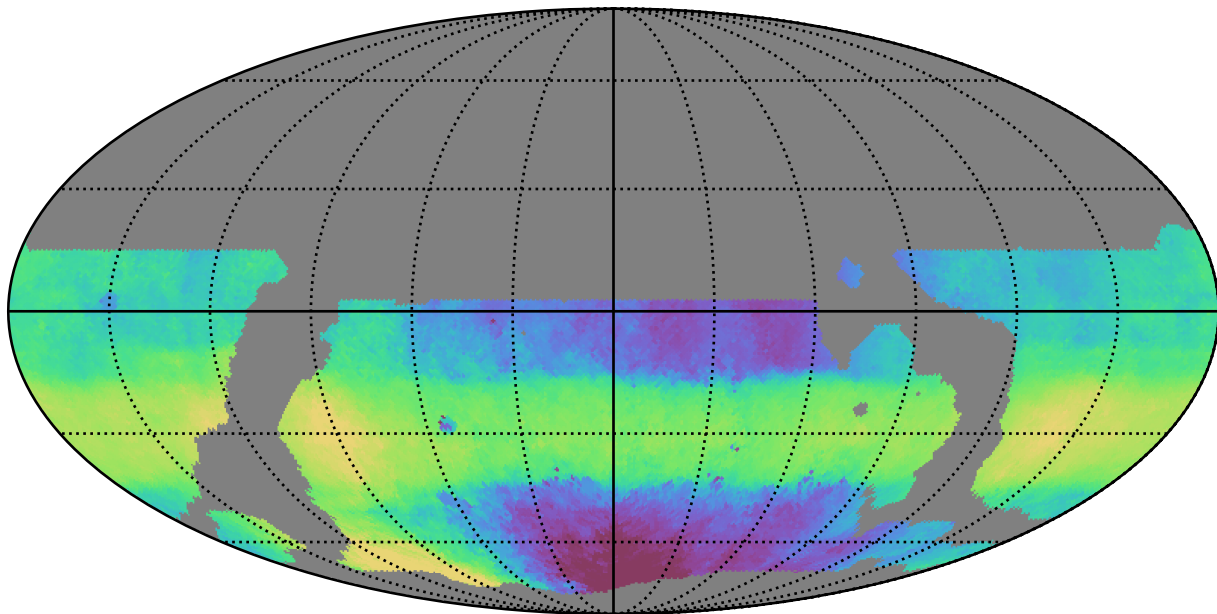
weather_cloudso18v3.4_10yrs WFD i band: Median HA
