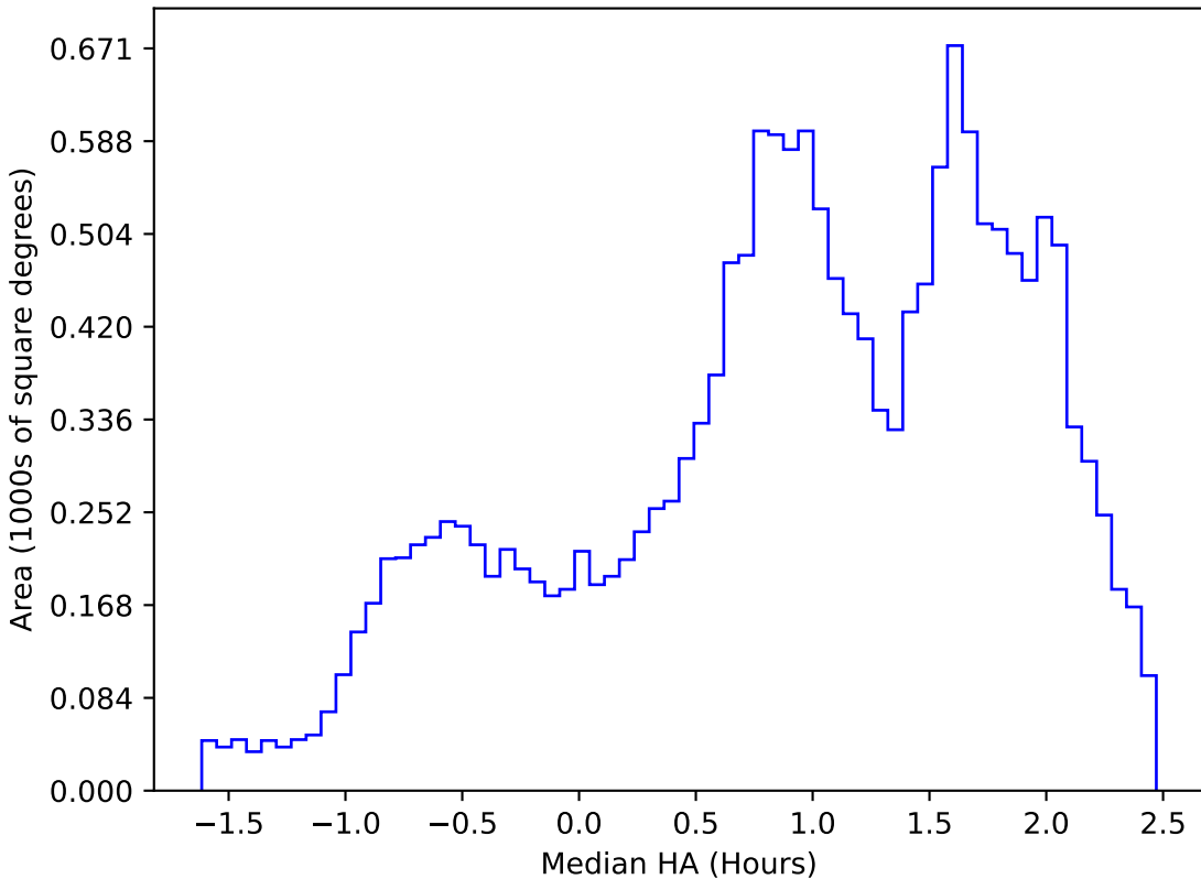
weather_cloudso18v3.4_10yrs WFD i band: Median HA
