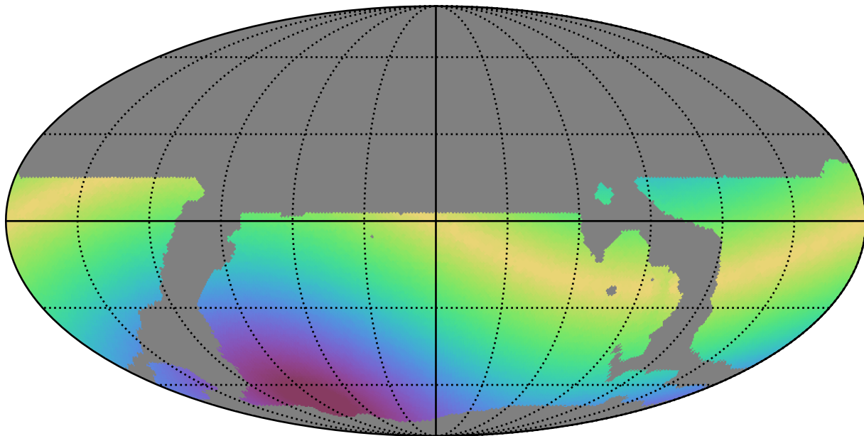
weather_cloudso18v3.4_10yrs WFD z band: Max solarElong
