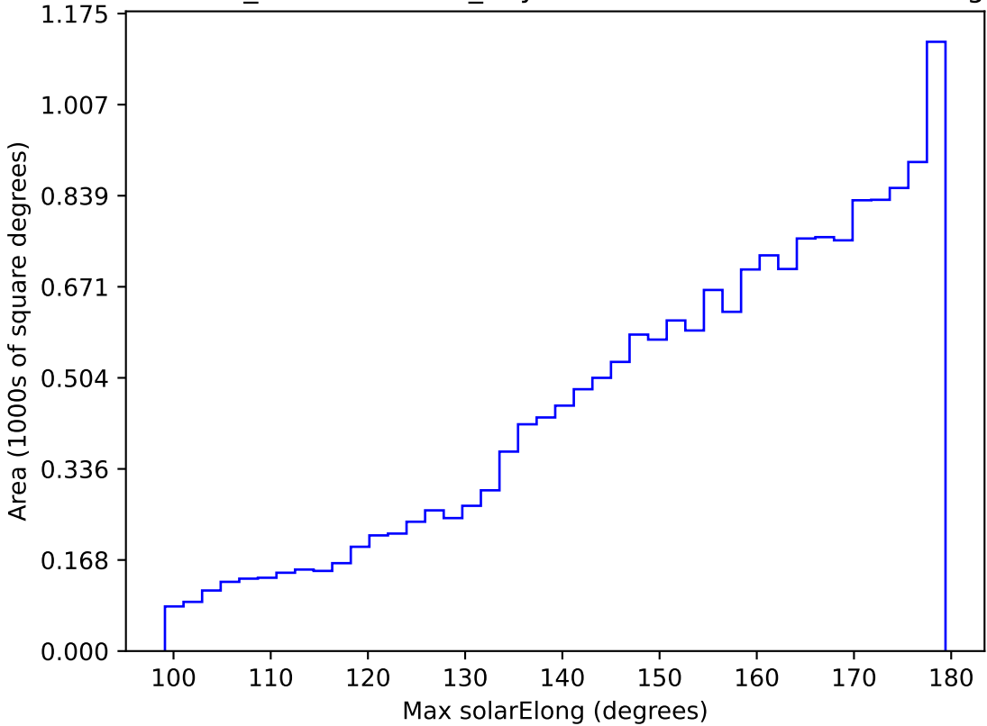
weather_cloudso18v3.4_10yrs WFD z band: Max solarElong
