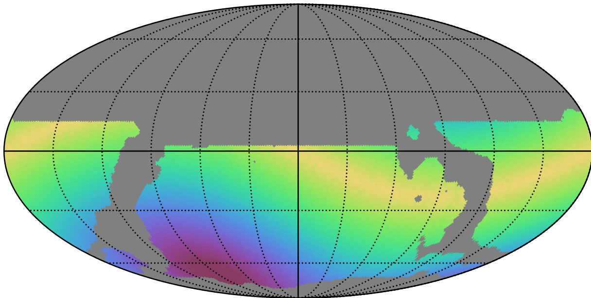
weather_cloudso18v3.4_10yrs WFD y band: Max solarElong
