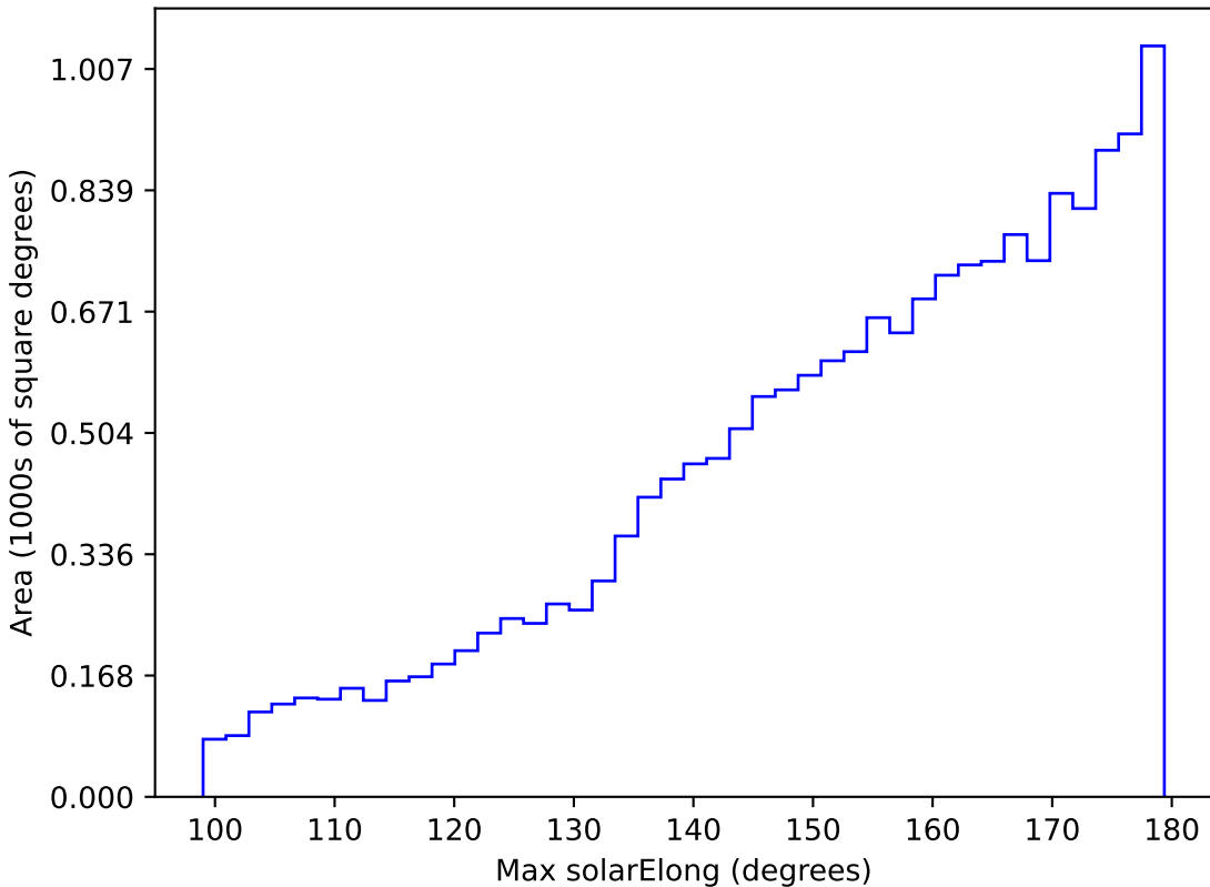
weather_cloudso18v3.4_10yrs WFD y band: Max solarElong
