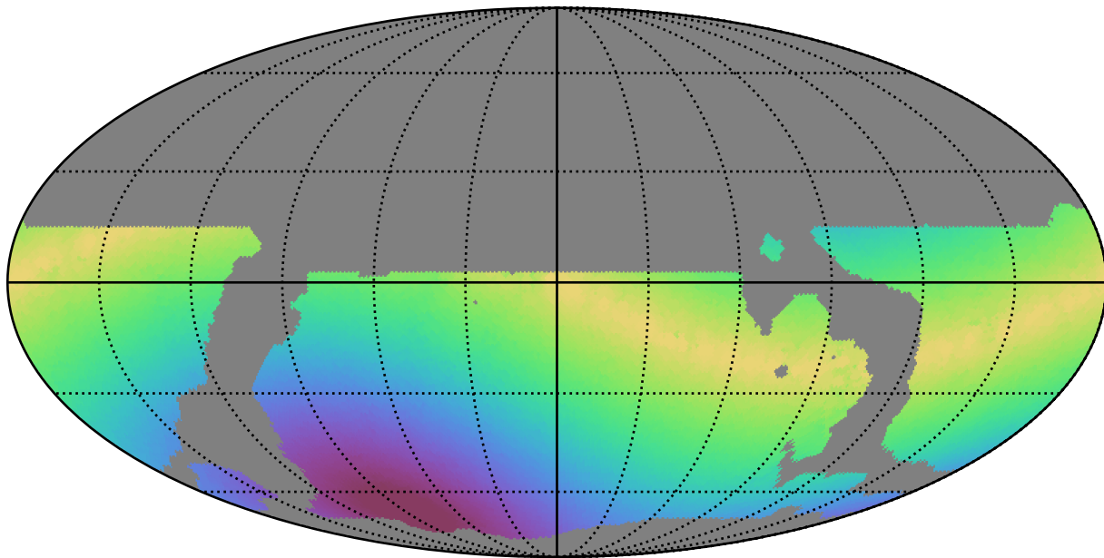
weather_cloudso18v3.4_10yrs WFD u band: Max solarElong
