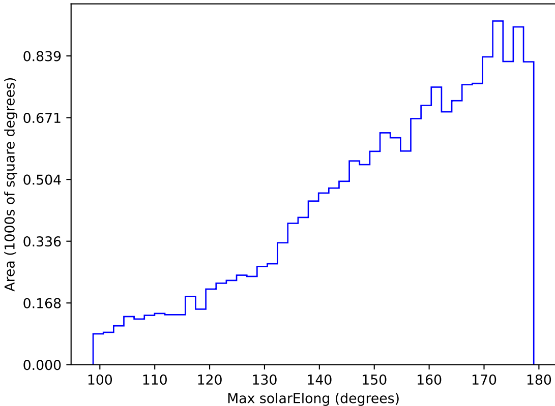
weather_cloudso18v3.4_10yrs WFD u band: Max solarElong
