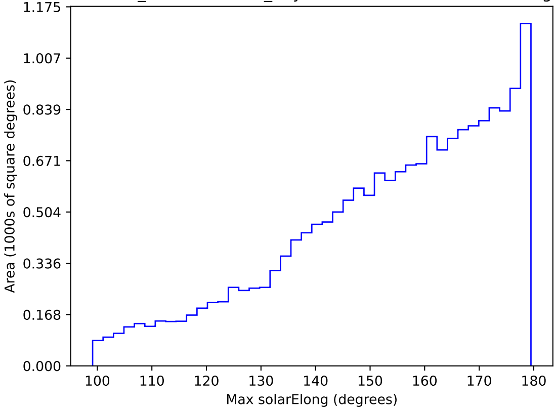
weather_cloudso18v3.4_10yrs WFD r band: Max solarElong
