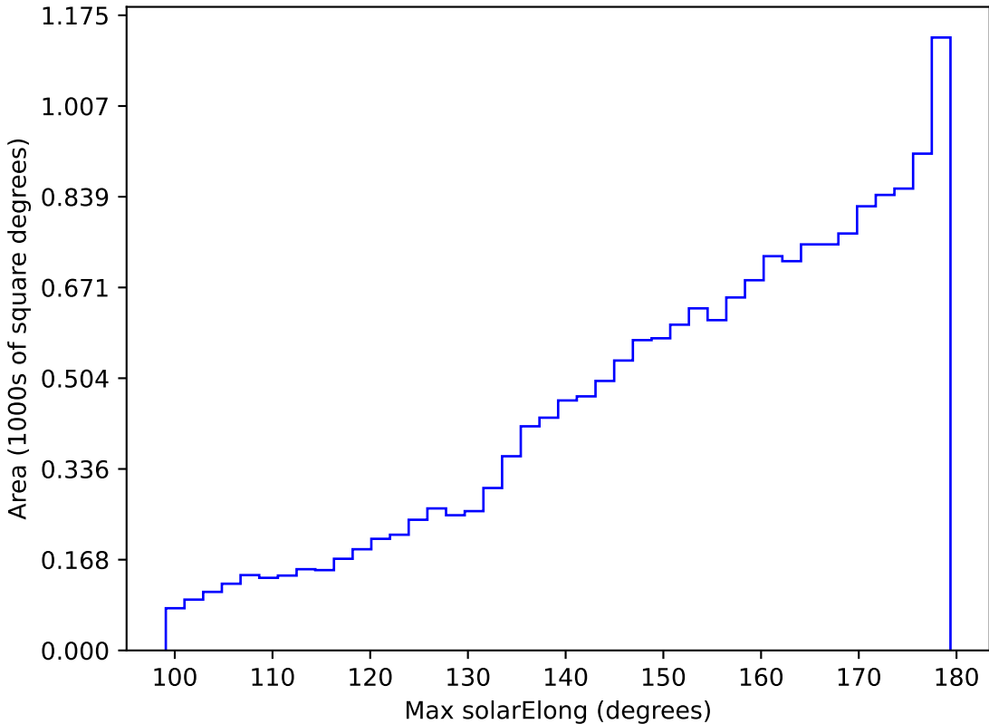
weather_cloudso18v3.4_10yrs WFD i band: Max solarElong
