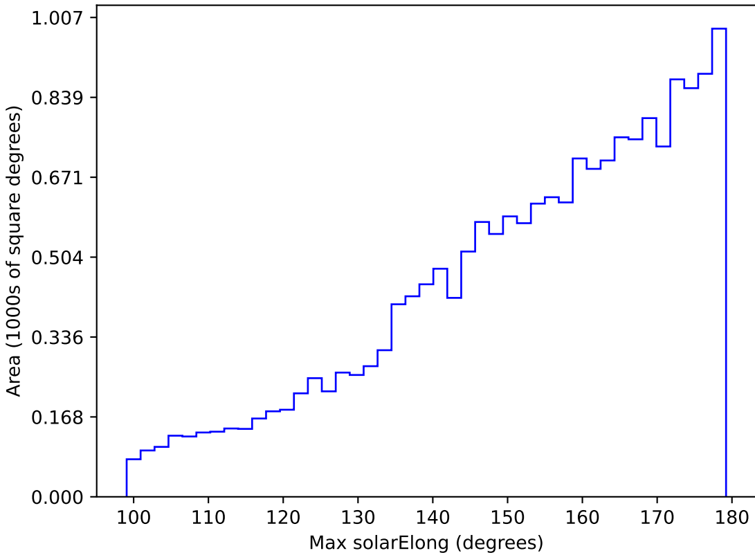
weather_cloudso18v3.4_10yrs WFD g band: Max solarElong
