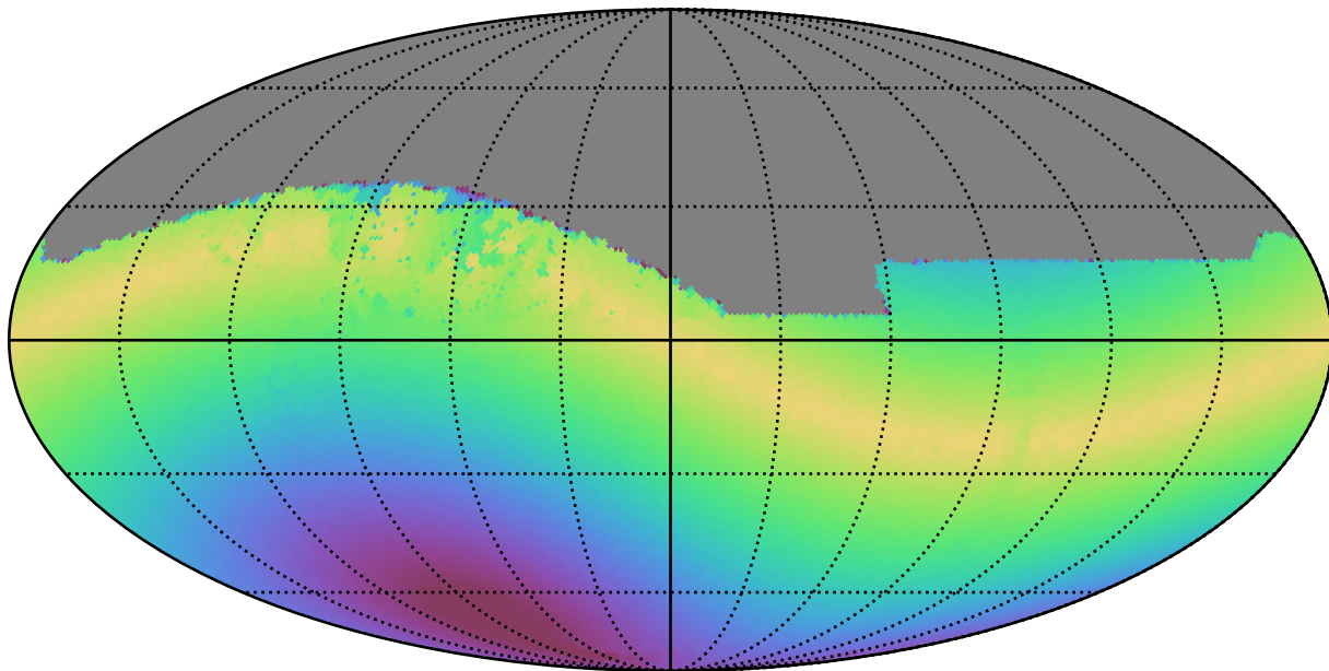
weather_cloudso18v3.4_10yrs All sky z band: Max solarElong
