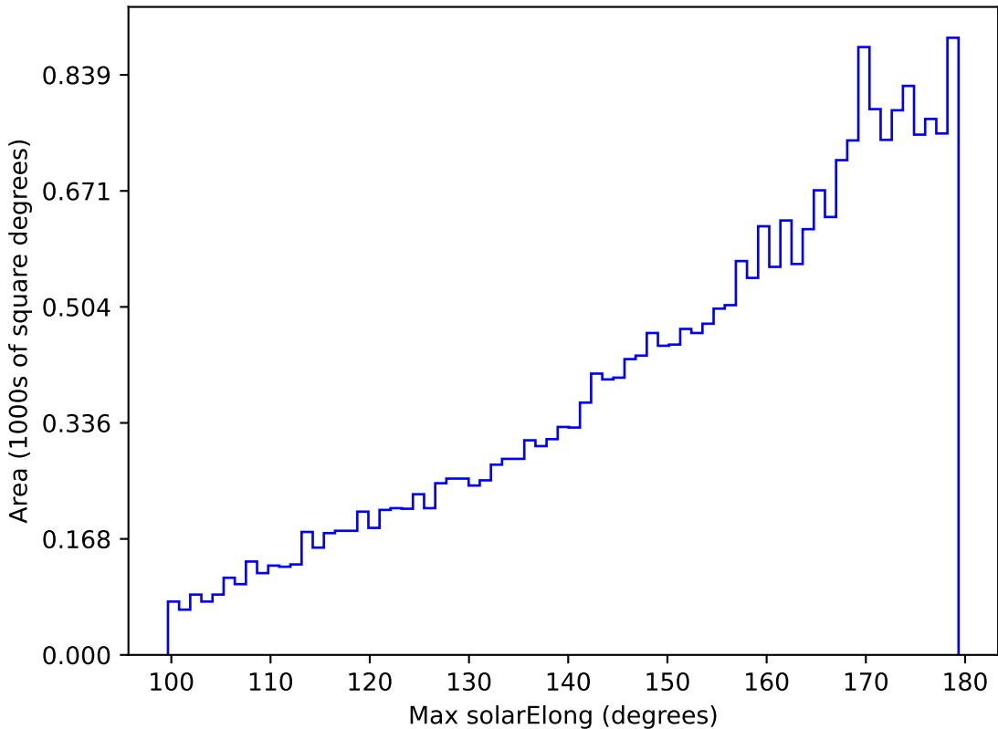
weather_cloudso18v3.4_10yrs All sky z band: Max solarElong
