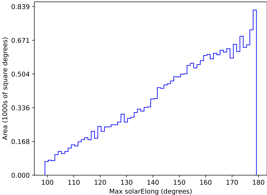
weather_cloudso18v3.4_10yrs All sky y band: Max solarElong
