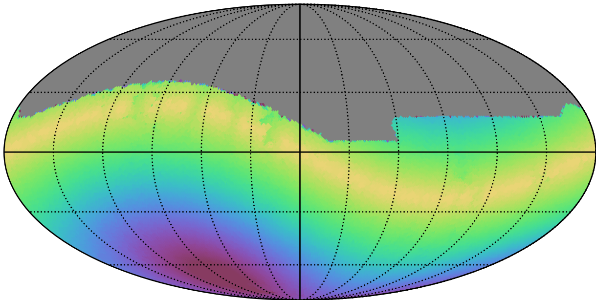
weather_cloudso18v3.4_10yrs All sky g band: Max solarElong
