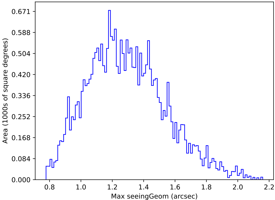
weather_cloudso18v3.4_10yrs Yr 1 z band: Max seeingGeom
