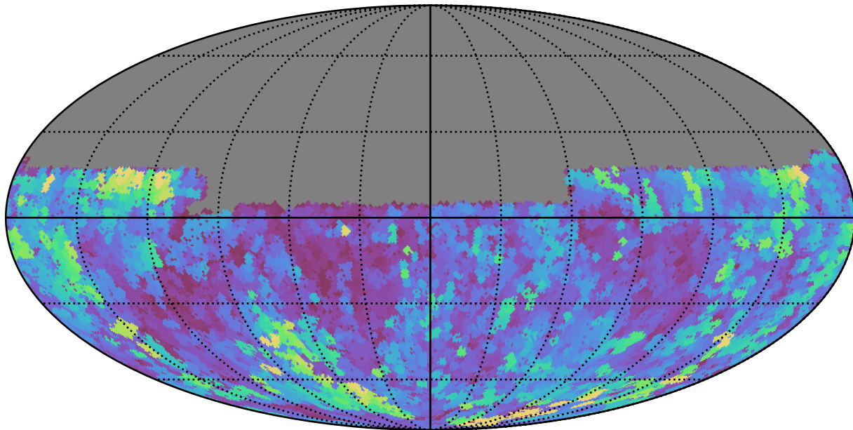
weather_cloudso18v3.4_10yrs Yr 1 y band: Max seeingGeom
