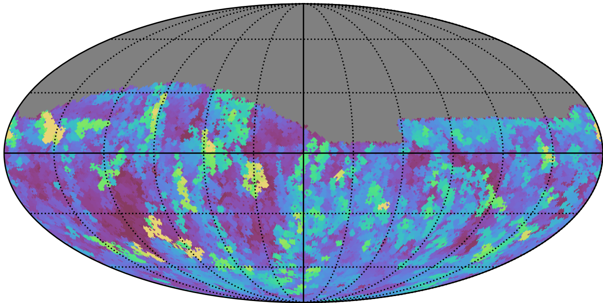
weather_cloudso18v3.4_10yrs Yr 1 i band: Max seeingGeom
