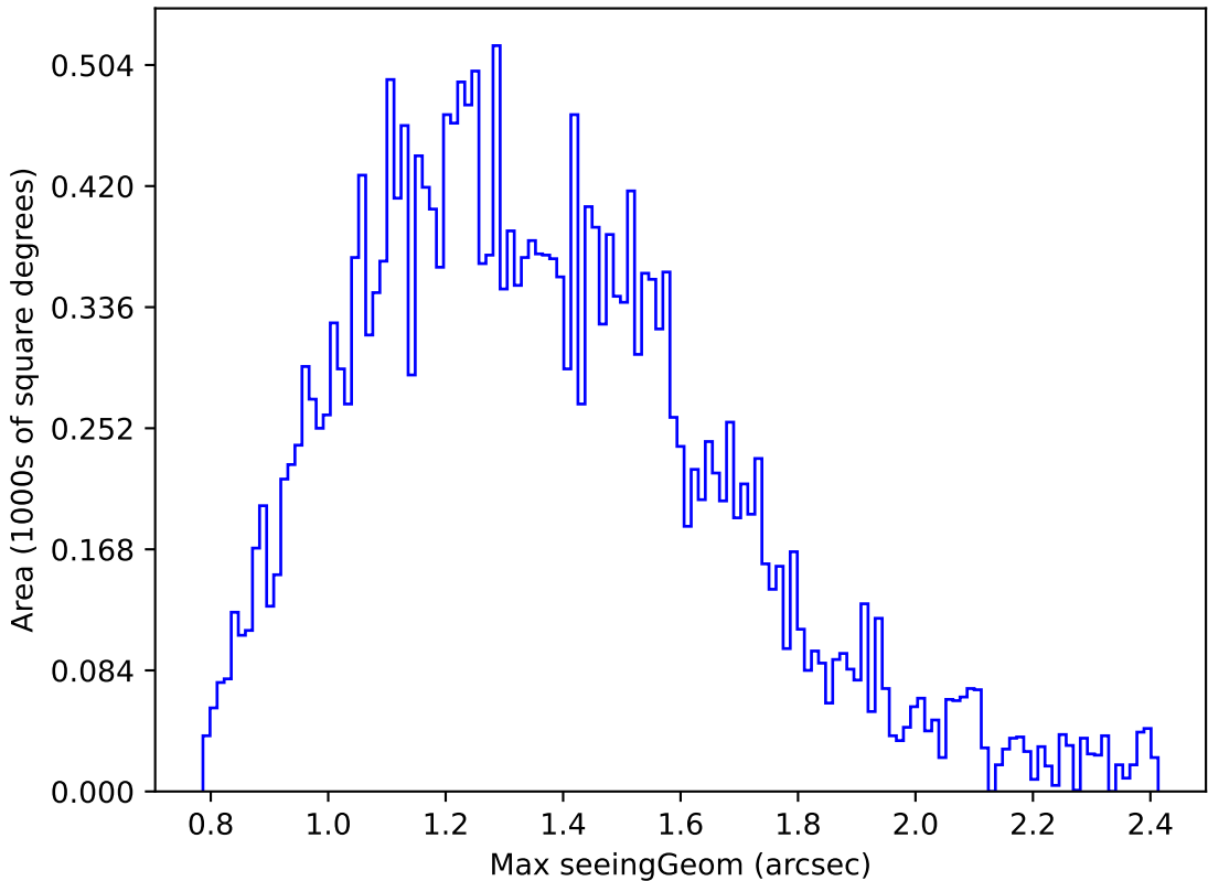
weather_cloudso18v3.4_10yrs Yr 1 i band: Max seeingGeom
