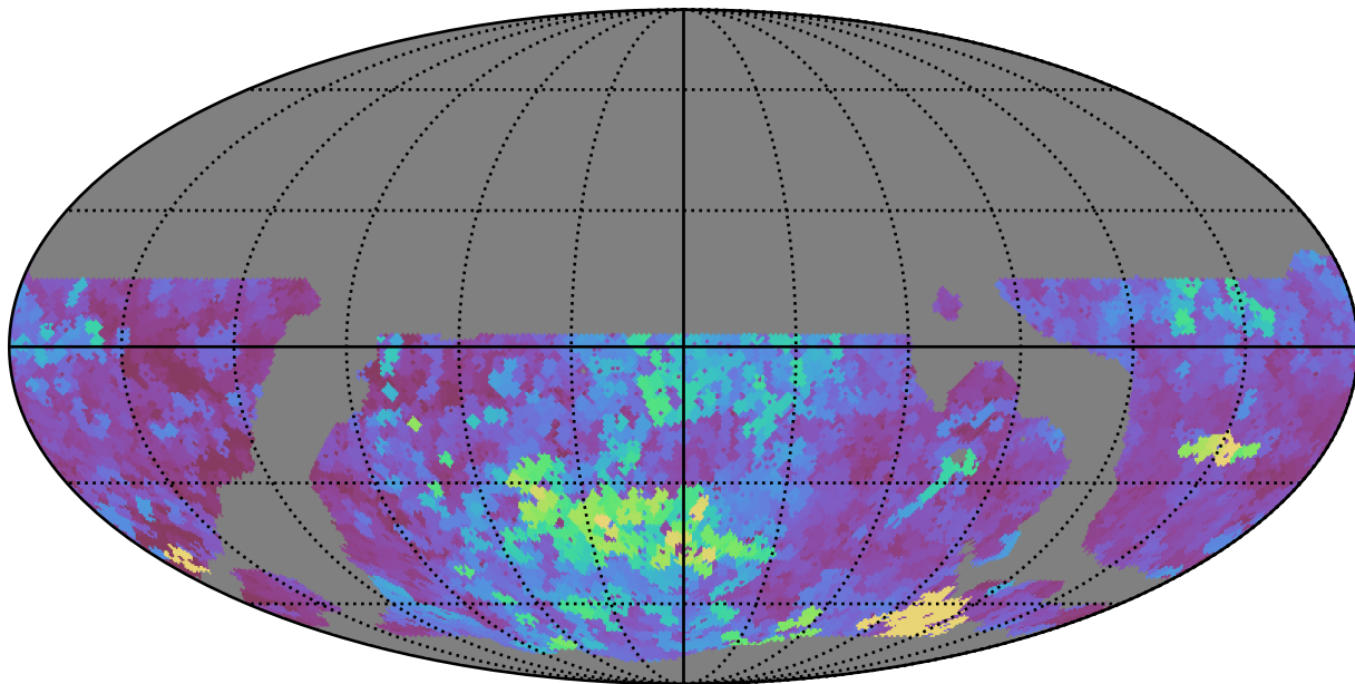
weather_cloudso18v3.4_10yrs WFD y band: Max seeingEff
