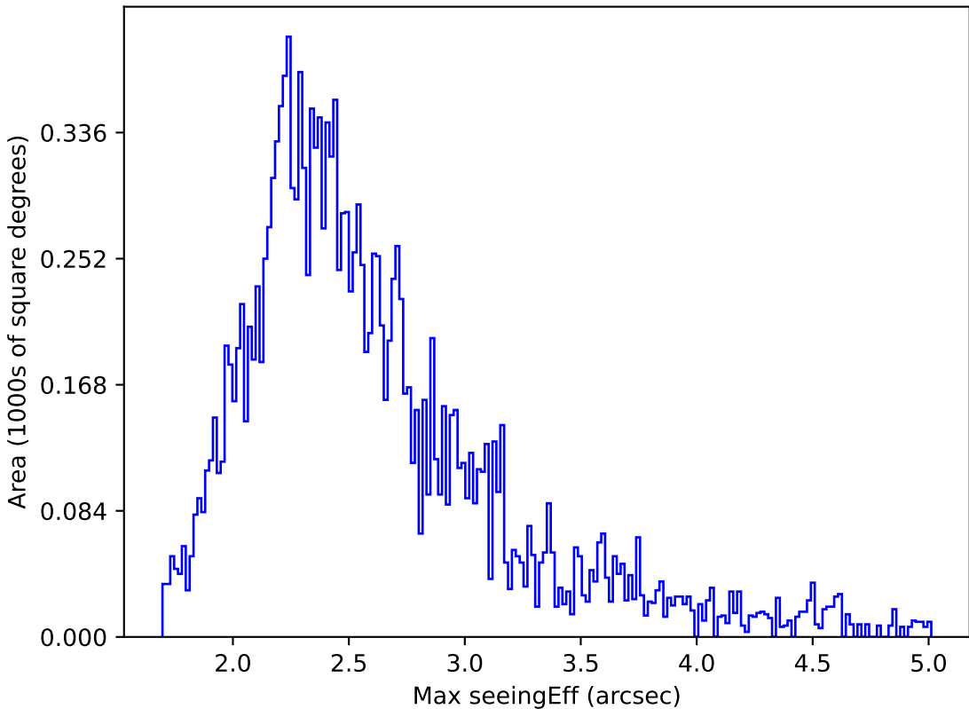
weather_cloudso18v3.4_10yrs WFD y band: Max seeingEff
