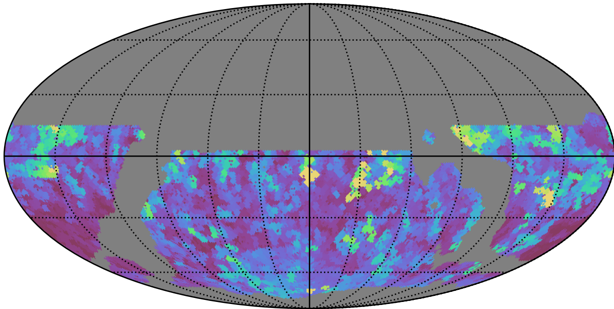
weather_cloudso18v3.4_10yrs WFD i band: Max seeingEff
