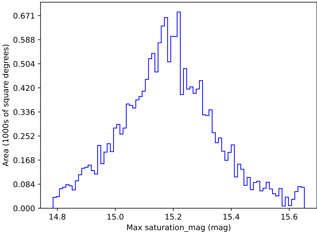
weather_cloudso18v3.4_10yrs WFD z band: Max saturation_mag
