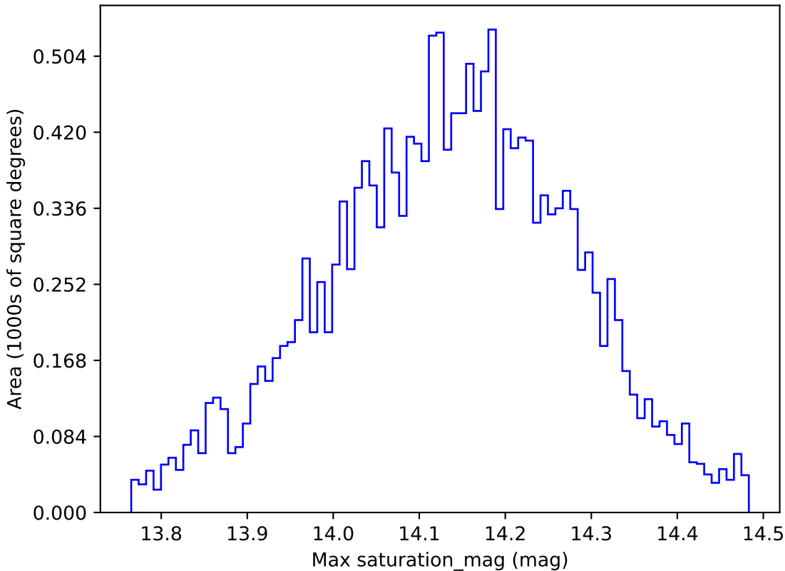
weather_cloudso18v3.4_10yrs WFD y band: Max saturation_mag
