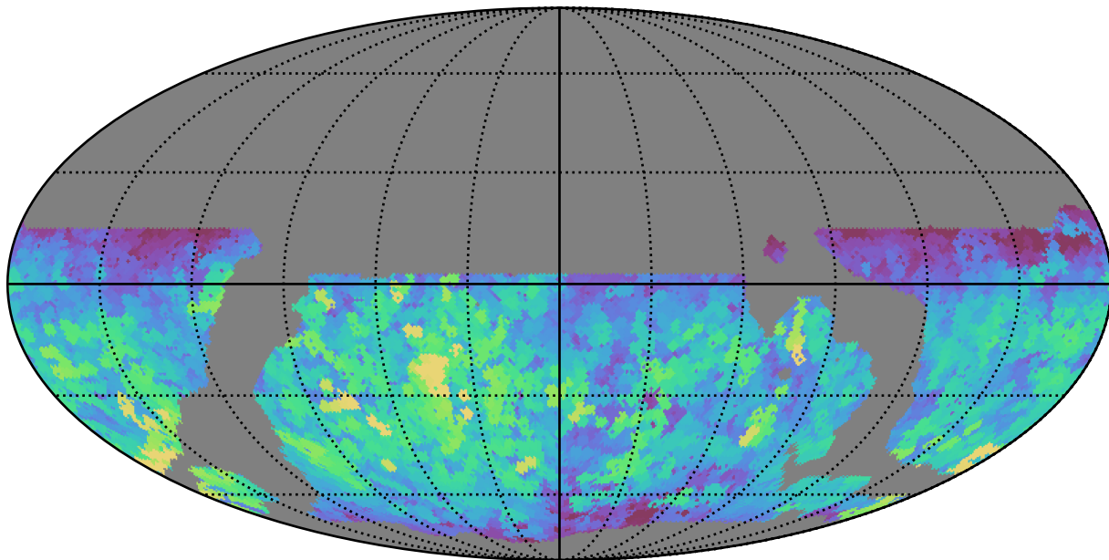
weather_cloudso18v3.4_10yrs WFD r band: Max saturation_mag
