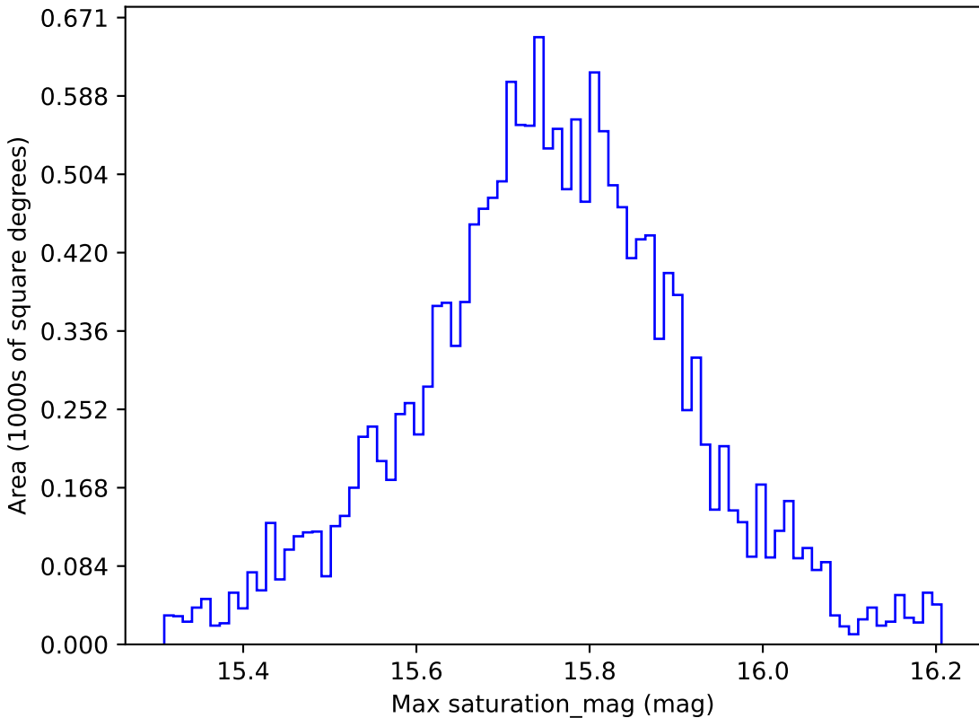
weather_cloudso18v3.4_10yrs WFD r band: Max saturation_mag
