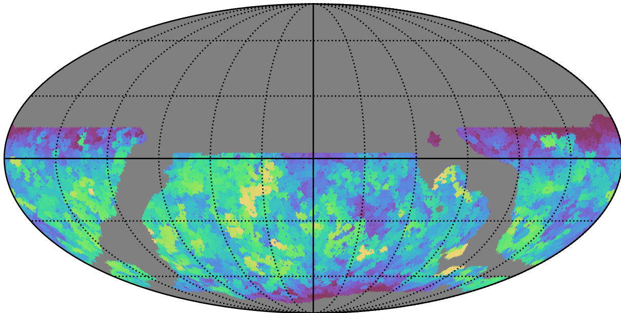
weather_cloudso18v3.4_10yrs WFD i band: Max saturation_mag
