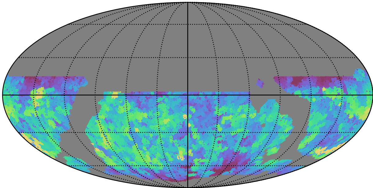
weather_cloudso18v3.4_10yrs WFD g band: Max saturation_mag
