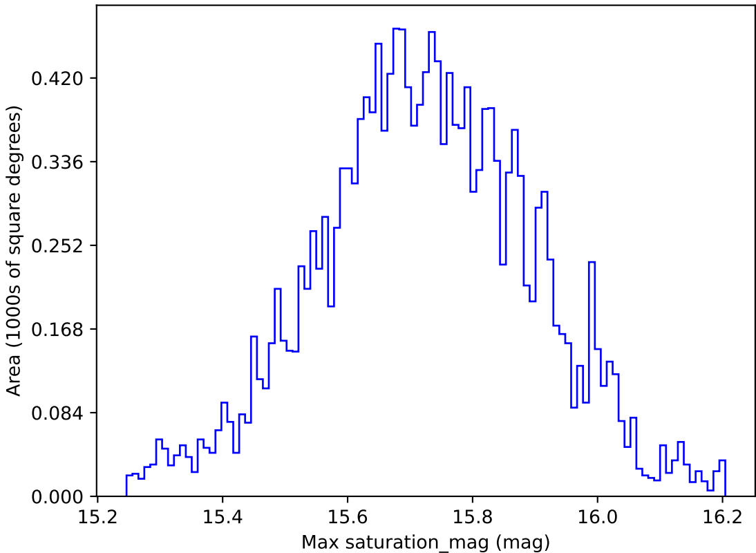
weather_cloudso18v3.4_10yrs WFD g band: Max saturation_mag
