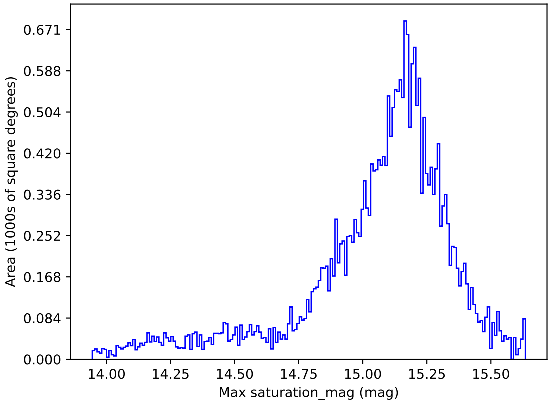
weather_cloudso18v3.4_10yrs All sky z band: Max saturation_mag
