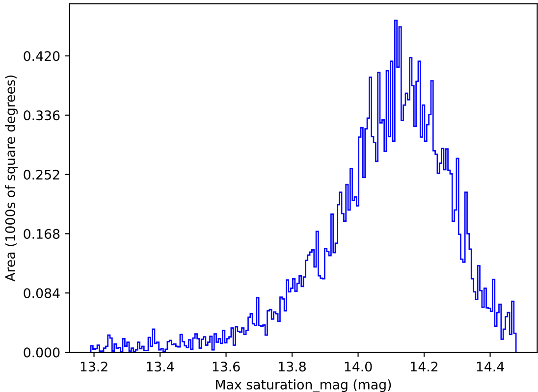
weather_cloudso18v3.4_10yrs All sky y band: Max saturation_mag
