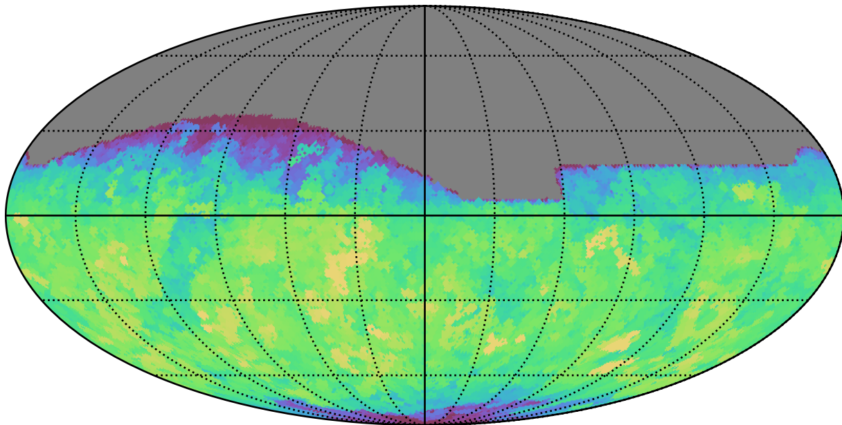
weather_cloudso18v3.4_10yrs All sky i band: Max saturation_mag
