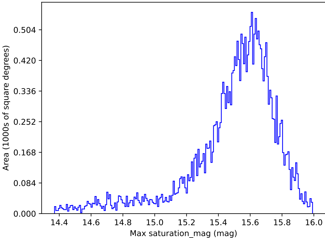
weather_cloudso18v3.4_10yrs All sky i band: Max saturation_mag
