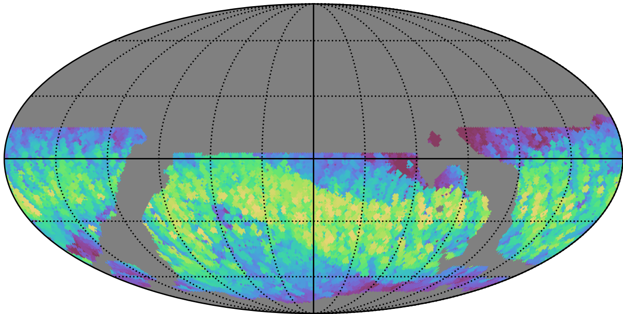
weather_cloudso18v3.4_10yrs WFD z band: Max normairmass
