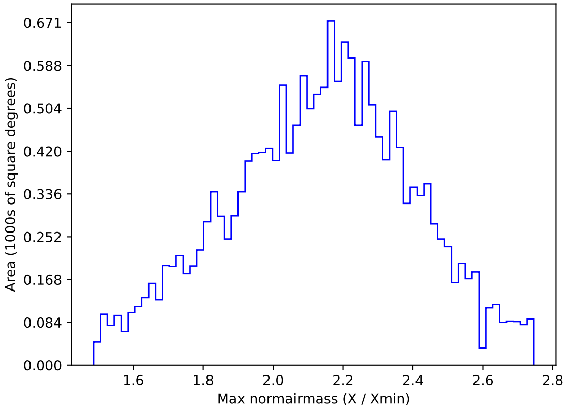
weather_cloudso18v3.4_10yrs WFD y band: Max normairmass
