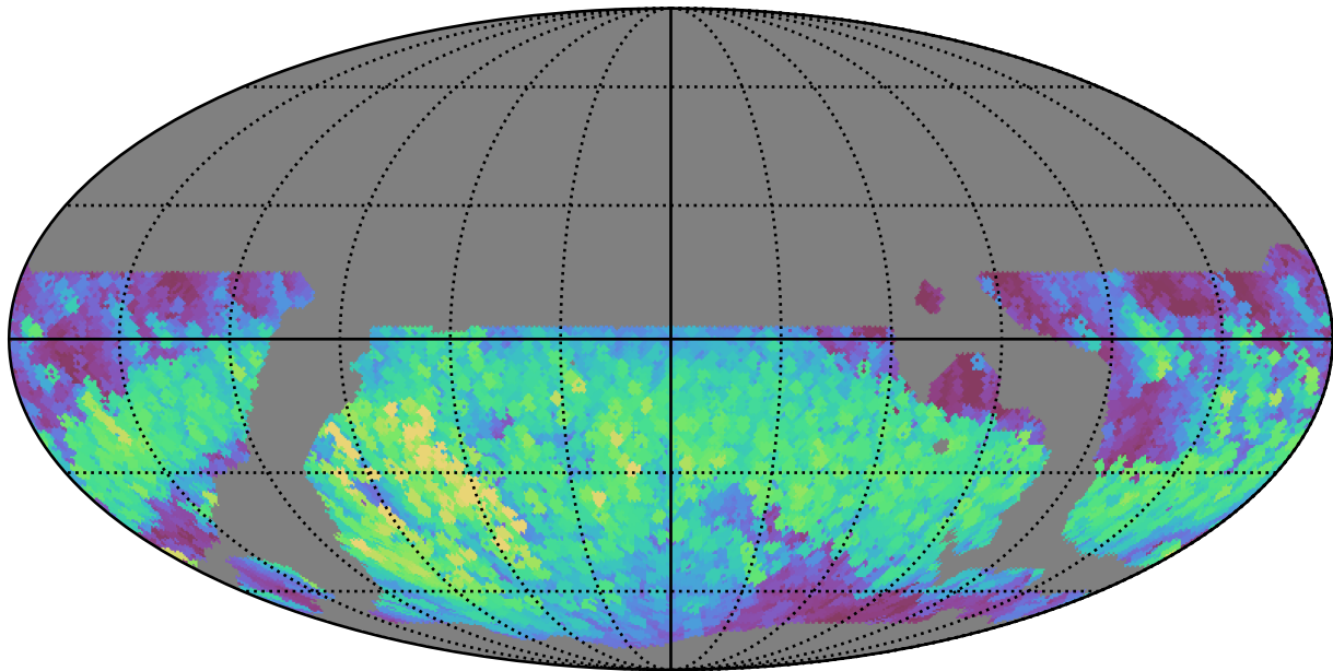
weather_cloudso18v3.4_10yrs WFD r band: Max normairmass
