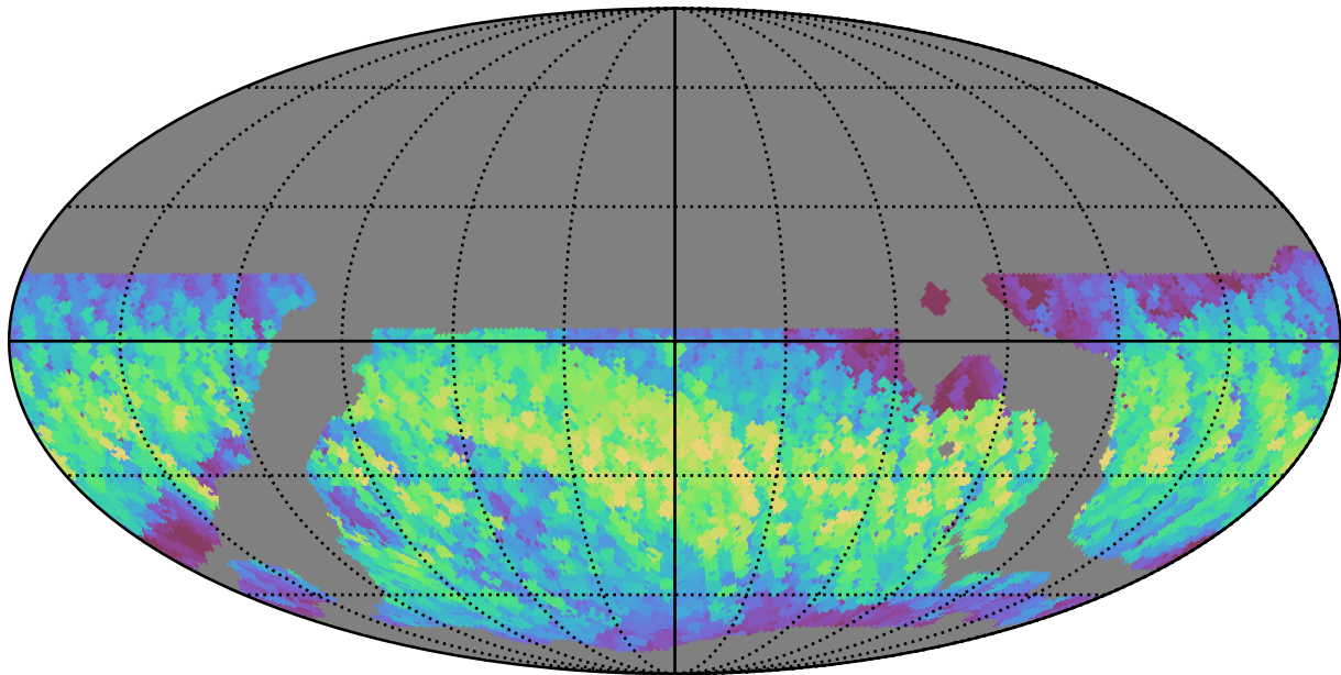
weather_cloudso18v3.4_10yrs WFD i band: Max normairmass
