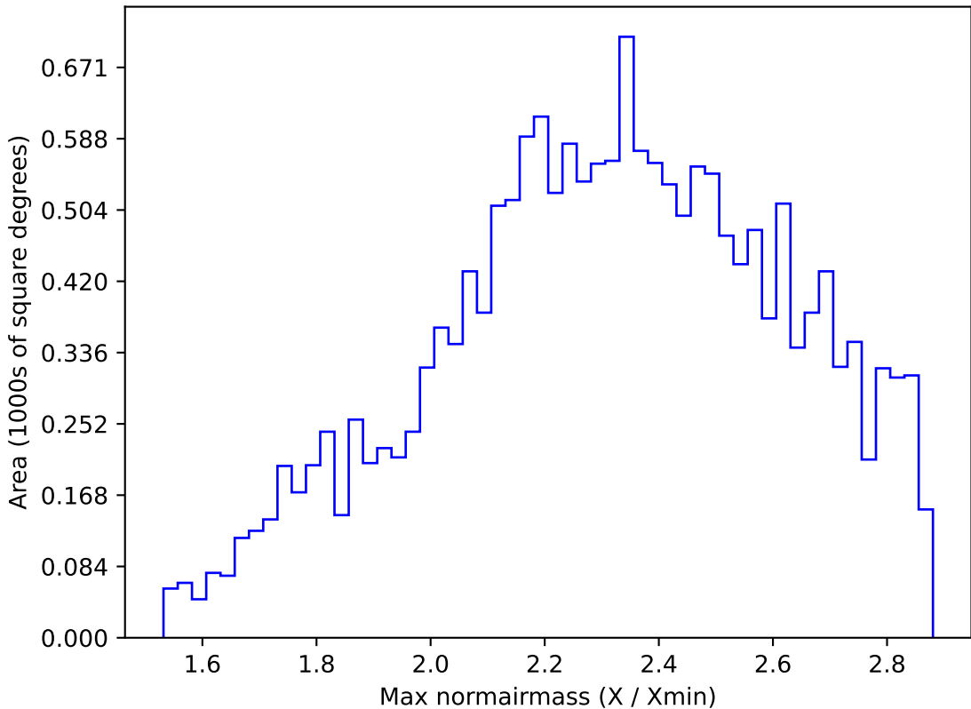
weather_cloudso18v3.4_10yrs WFD i band: Max normairmass
