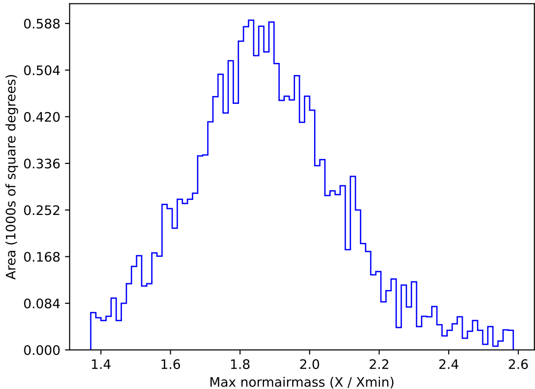
weather_cloudso18v3.4_10yrs WFD g band: Max normairmass
