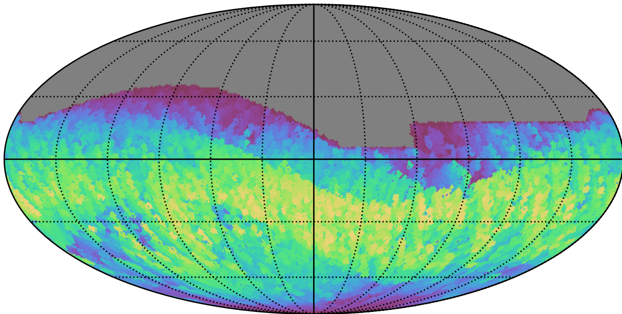
weather_cloudso18v3.4_10yrs All sky z band: Max normairmass
